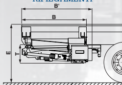
MOTRICE - PIANALE 2 RIPIEGAMENTI
