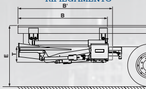
MOTRICE - PIANALE 1 RIPIEGAMENTO
