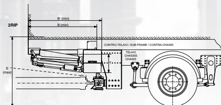
MOTRICE - PIANALE 2 RIEPIEGAMENTI
