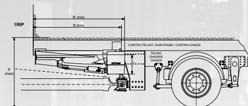
MOTRICE - PIANALE 1 RIEPIEGAMENTO
