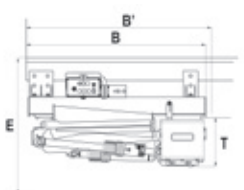
MONTAJE LATERAL PARA MÁQUINAS MOTRICES PLATO 2 PLEGADOS
