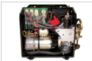
Grupo hidráulico
