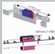
33 F3CL080 - Centralita hidráulica colocada centralmente para acabados de anchura reducida.
