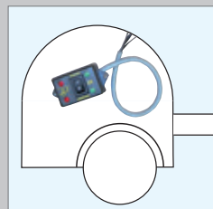
40 Interruptor en cabina con indicadores luminosos para: puesta en marcha o apagado de la trampilla, plataforma abierta.
