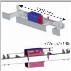
34 F3CL10 - Centralita hidráulica colocada centralmente para acabados de anchura reducida.
